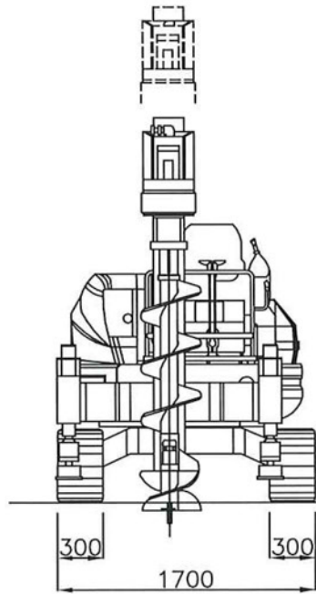
正面図
