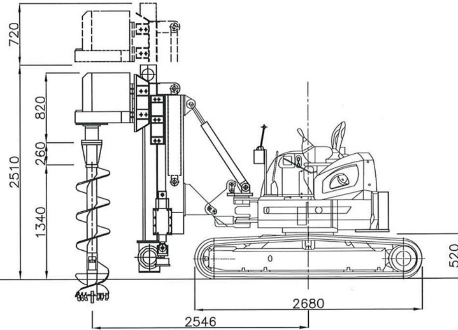
側面図
